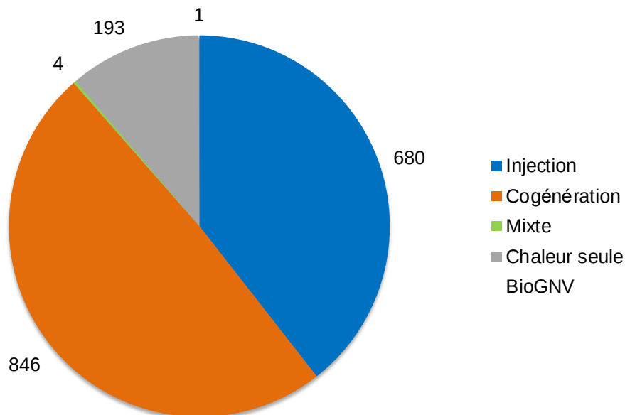
Répartition des unités par type de valorisation
