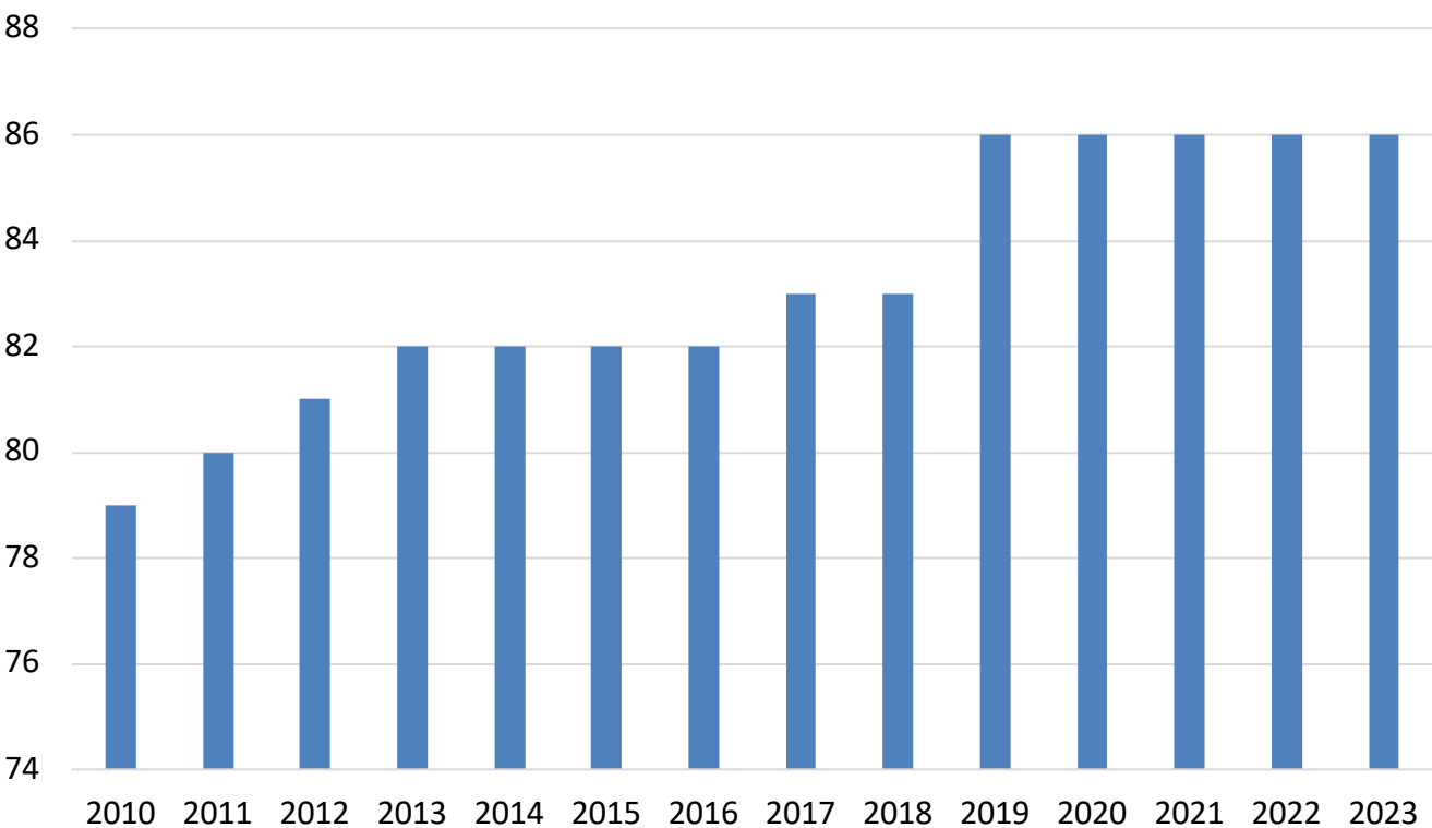
Evolution du parc de méthanisation d'industrie Valorisation chaleur seule (en nbre d'unités)
